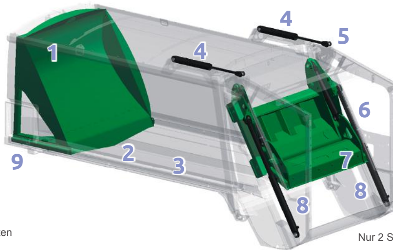
8 Außenliegende Zylinder
