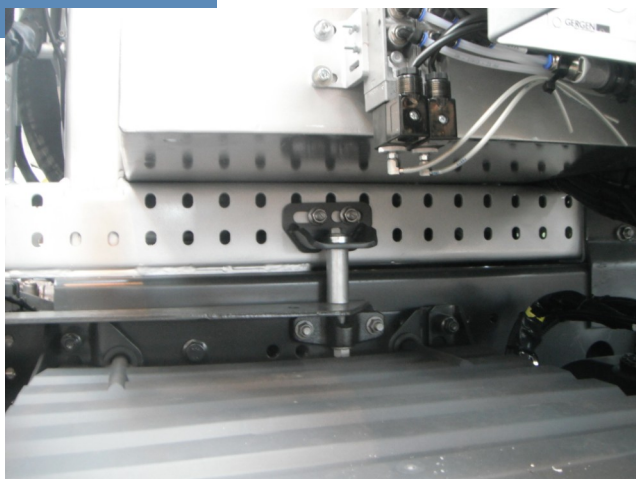
Schweißfreie Montage
