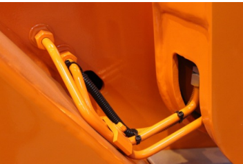
Wenig Einsatz von Hydraulikschläuchen, verschleißarme Verlegung
