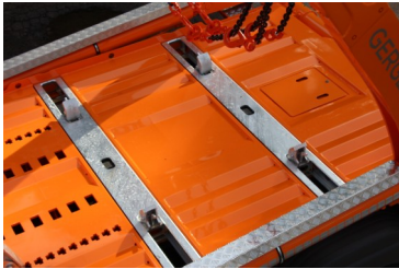
4fach hydraulische Behälterverriegelung feuerverzinkt
